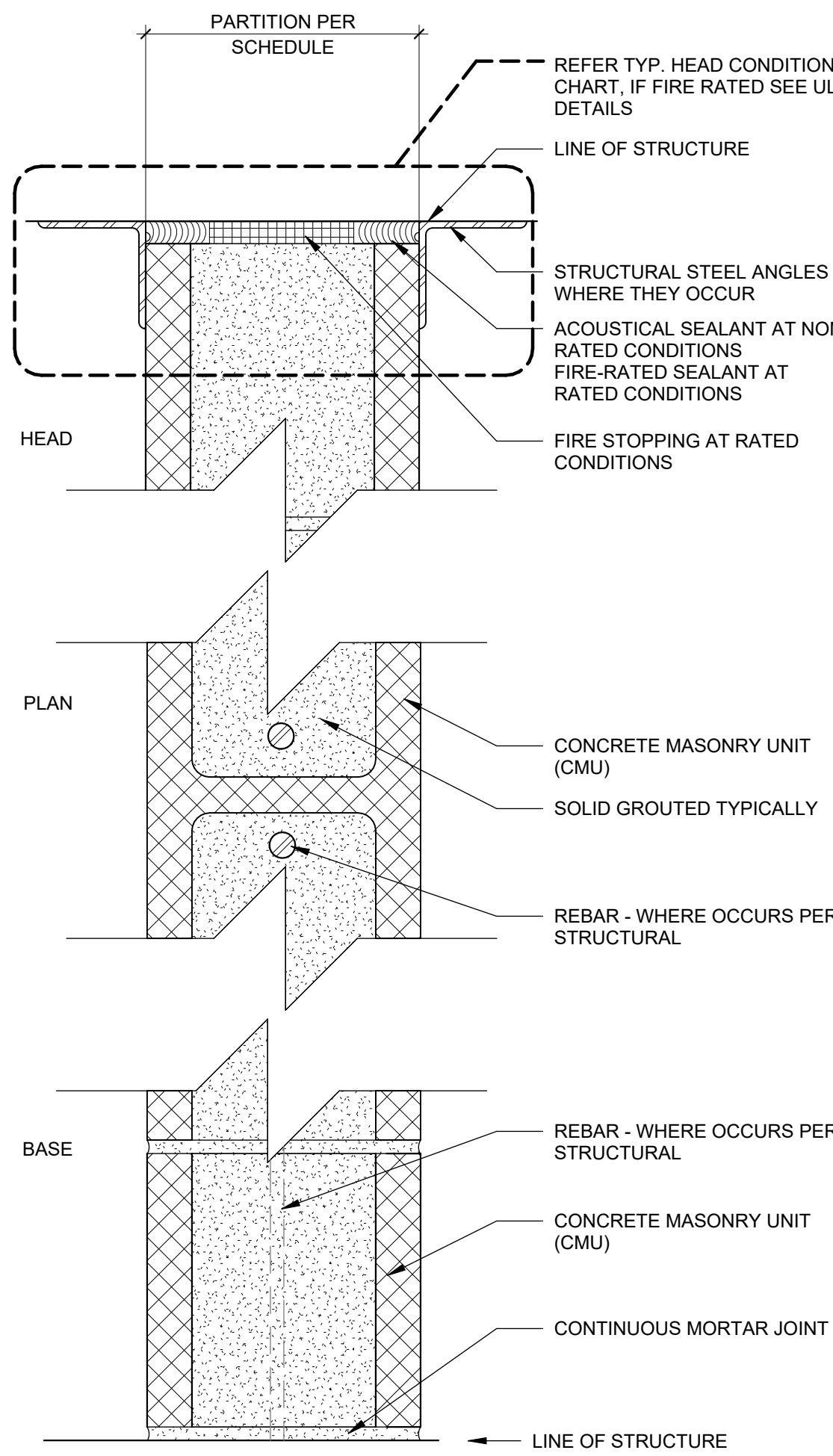
4 M TYPE PARTITION N.T.S.
