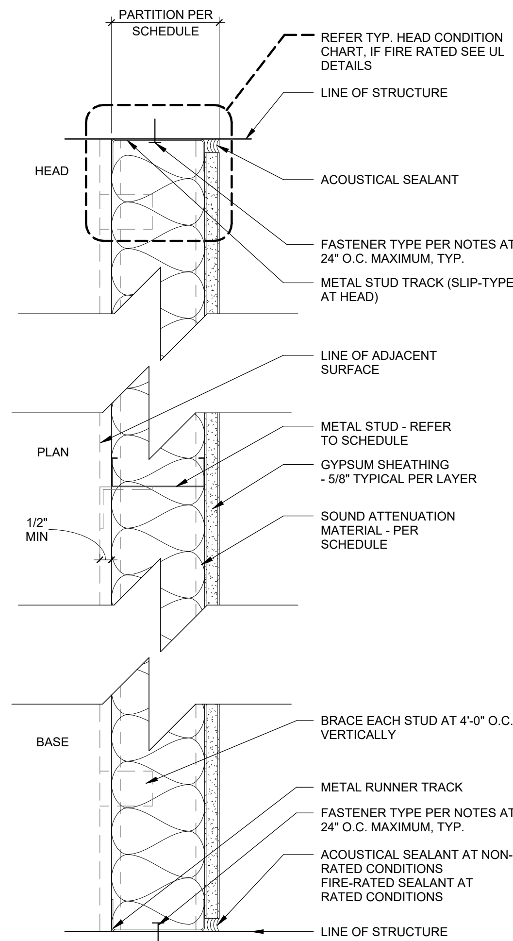
2 H TYPE PARTITION N.T.S.
