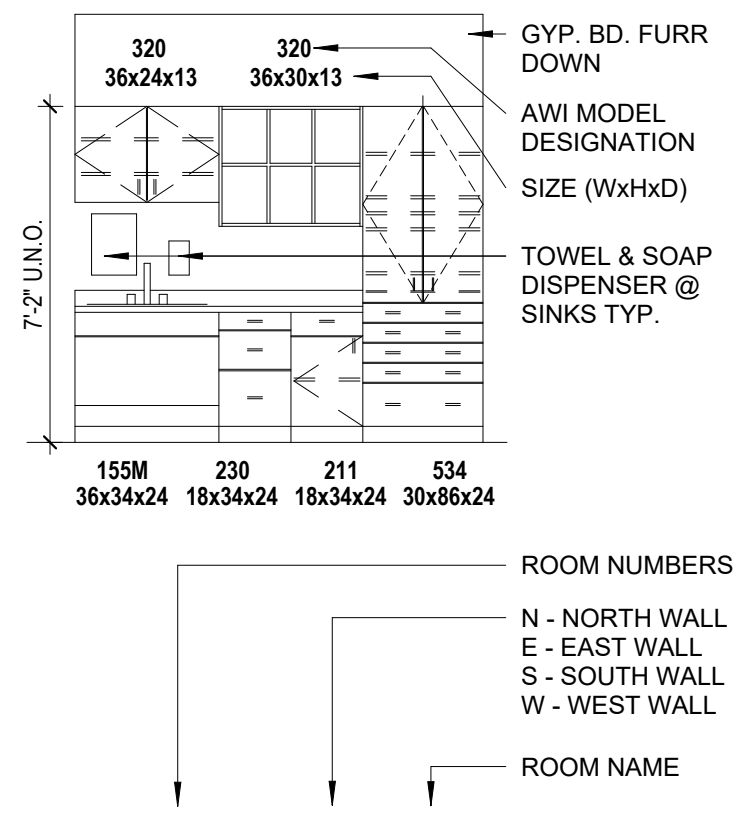
01 1120 - E BREAK 1/4" = 1'-0"
