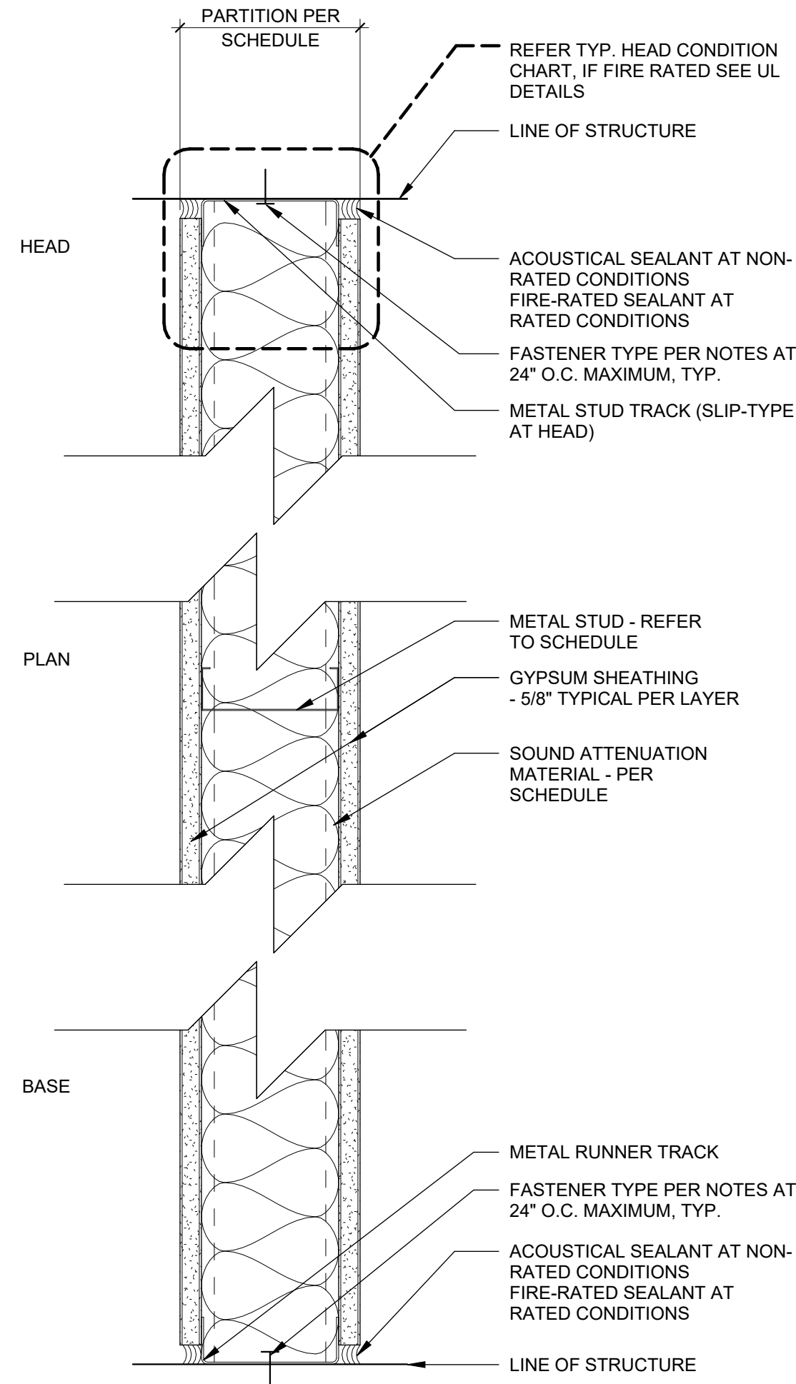
1 A TYPE PARTITION N.T.S.
