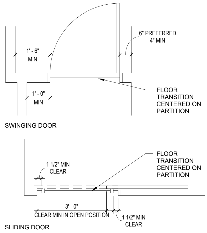
DOOR CLEARANCE DIAGRAMS
